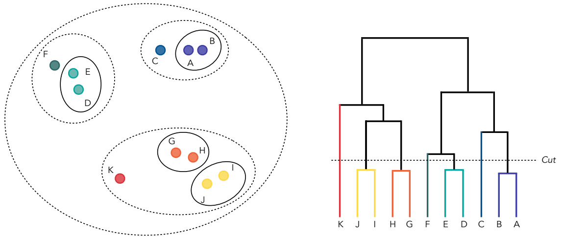
Figure 4.3 – Exemple de regroupement hiérarchique et de dendrogramme
