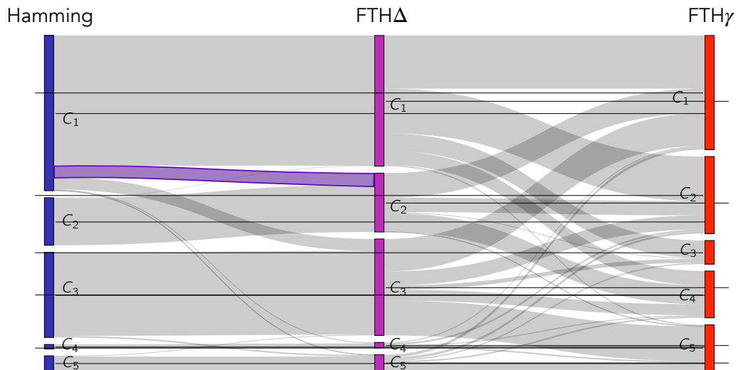
Figure 6.8 – Diagramme de Sankey illustrant les flux entre les 3 partitions formées par les mesures de Hamming, FTH\Delta et FTH\gamma
