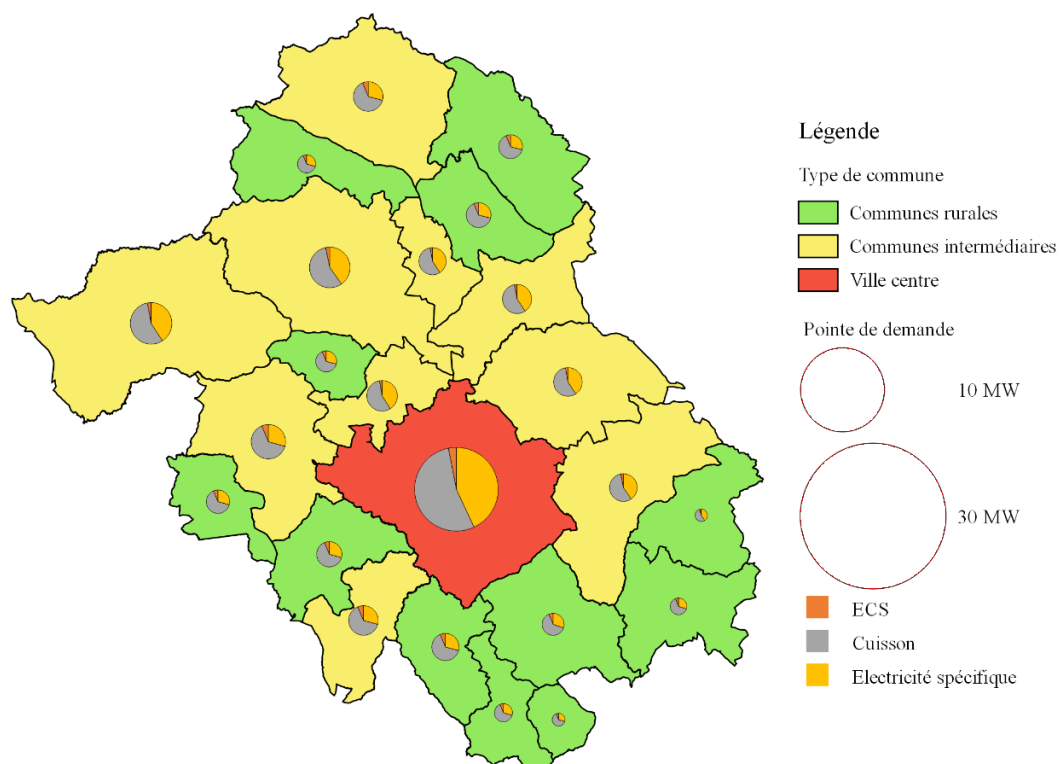
Figure 81: Pointe de demande électrique selon les usages pour le scénario Volontariste 2050
