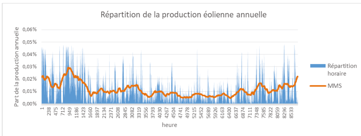
Figure 72: Courbe de répartition de la production éolienne (d'après Eco2mix 2016)
