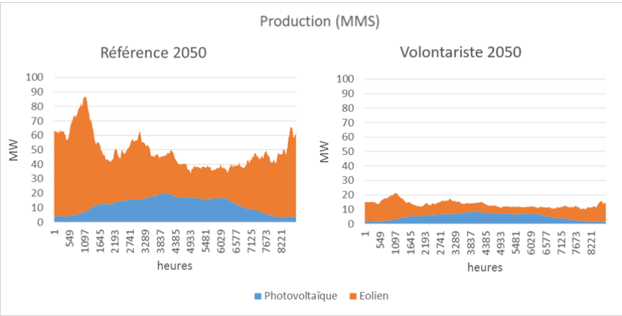
Figure 95: Variations saisonnières de la production électrique par filière selon les scénarios
