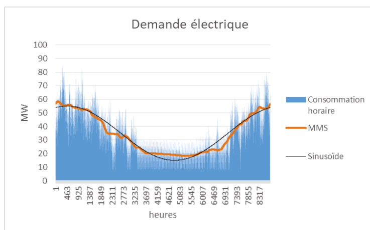
Figure 49: Variations horaire et saisonnière de la demande électrique résidentielle du Pays Yon et Vie en 2015 42
