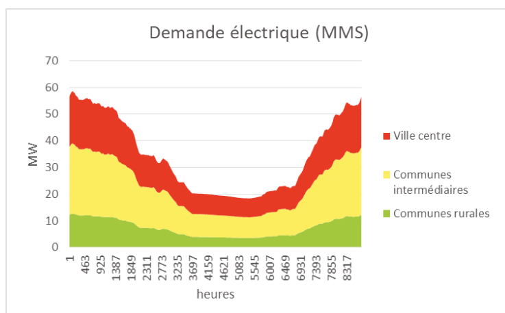
Figure 51: Variations saisonnières de la demande électrique résidentielle du Pays Yon et Vie selon la typologie de communes en 2015
