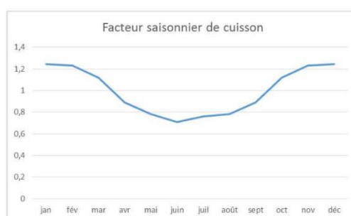
Figure 106: Facteur saisonnier de consommation énergétique de cuisson (d'après Sidler 1999)
