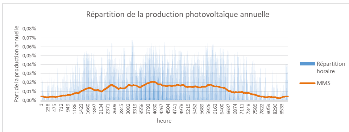
Figure 71: Courbe de répartition de la production photovoltaïque (d'après Eco2mix 2016)
