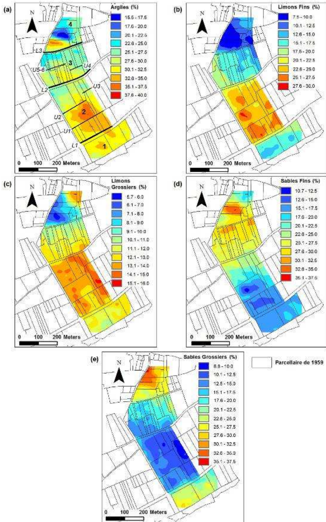
Figure V-5. Distribution spatiale de la granularité de l'horizon superficiel (0-20 cm) par krigeage ordinaire sur l'échantillonnage \Delta : (a) argiles A (< 2 μm), (b) limons fins LF (2-20 μm), (c) limons grossiers LG (20-50 μm), (d) sables fins SF (50-200 μm) et (e) sables grossiers SG (200 μm - 2 mm). L1 à L3 : banquettes agricoles ; U1 à U5-6 : ondulations ; 1 à 4 : unités morphologiques.
